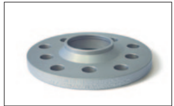
Artikel-Nr./Part-no. 24255570A: Radnabellänge max. 17 mm. Felgeninnenfase mind. 7x45° Wheel hub length max. 17 mm. Inner bavel 7x45°.
