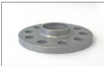
Artikel-Nr./Part-no. 2025541: Radnabenlänge max. 10 mm. Wheel hub length max. 10 mm.
