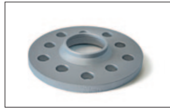
Artikel-Nr./Part-no. 2055573A, 2055577A: Radnabenlänge max. 15 mm. Felgeninnenfase mind. 6x45° Wheel hub length max. 15 mm. Inner bavel 6x45°
