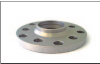
Artikel-Nr./Part-no. 2455571, 2455577: Radnabenlänge max. 15 mm. Felgeninnenfase mind. 5x45° Wheel hub length max. 15 mm. Inner bavel 5x45°.
