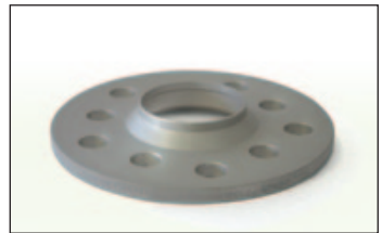
Artikel-Nr./Part-no. 1655572: Radnabellänge max. 14 mm. Felgeninnenfase mind. 7x45° Wheel hub length max. 14 mm. Inner bavel 7x45°.
