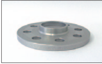
Artikel-Nr./Part-no. 20245414, 20245410, 202454101, 2024541: Radnabenlänge max. 11 mm. Wheel hub length max. 11 mm.
