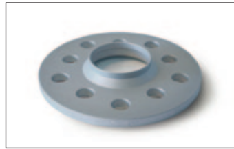
Artikel-Nr./Part-no. 1655573, 1655577: Radnabenlänge max. 12 mm. Felgeninnenfase mind. 6x45° Wheel hub length max. 12 mm. Inner bavel 6x45°
