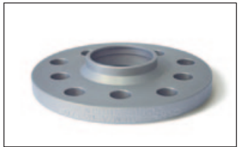
Artikel-Nr./Part-no. 24255570B: Radnabellänge max. 14,5 mm. Felgeninnenfase mind. 5x45° Wheel hub length max. 14,5 mm. Inner bavel 5x45°.
