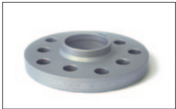
Artikel-Nr./Part-no. 30255570: Radnabellänge max. 17 mm. Felgeninnenfase mind. 4x45° Wheel hub length max. 17 mm. Inner bavel 4x45°.
