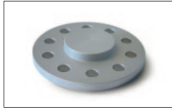
Artikel-Nr./Part-no. 22556659: Radnabenlänge max. 9 mm. Wheel hub length max. 9 mm.
