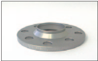
Artikel-Nr./Part-no. 162345712: Radnabellänge max. 14 mm. Felgeninnenfase mind. 7x45° Wheel hub length max. 14 mm. Inner bavel 7x45°.
