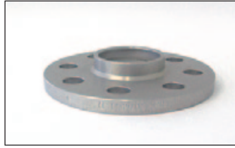
Artikel-Nr./Part-no. 20245616: Radnabenlänge max. 10 mm. Wheel hub length max. 10 mm.
