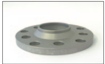
Artikel-Nr./Part-no. 202555712A: Radnabellänge max. 16 mm. Felgeninnenfase mind. 7x45° Wheel hub length max. 16 mm. Inner bavel 7x45°.
