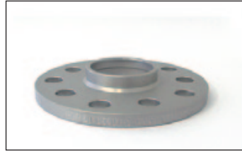
Artikel-Nr./Part-no. 20365601: Radnabenlänge max. 11 mm. Wheel hub length max. 11 mm.
