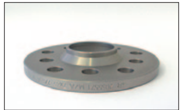
Artikel-Nr./Part-no. 2055571A: Radnabellänge max. 15,5 mm. Felgeninnenfase mind. 6,5x45° Wheel hub length max. 15,5 mm. Inner bavel 6,5x45°.
