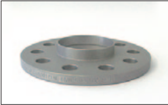
Artikel-Nr./Part-no. 2055665: Radnabenlänge max. 9 mm. Wheel hub length max. 9 mm.
