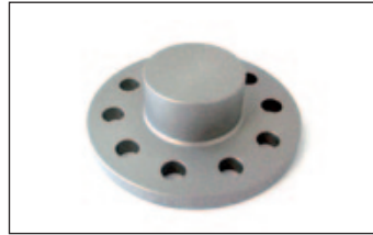
Artikel-Nr./Part-no. 20556659, 24556659, 30556659. Spezielle Aussenkantur für Daimler Chrysler-Modelle an der Vorderachse/ special outer contour for DaimlerChry- sler-cars on the front axle
