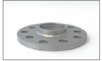
Artikel-Nr./Part-no. 20656014: Radnabenlänge max. 11 mm. Wheel hub length max. 11 mm.
