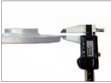
Darstellung Aussenfase 5x45°/Outer bavel 5x45°
