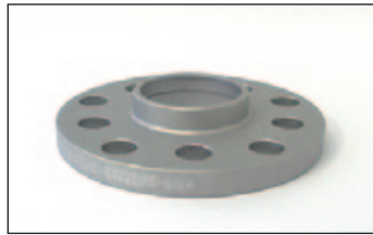
Artikel-Nr./Part-no. 24135580, 24135584: Radnabenlänge max. 12,5 mm. Wheel hub length max. 12,5 mm.
