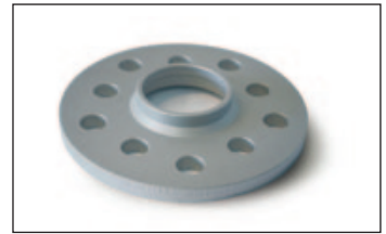
Artikel-Nr./Part-no. 2055573B, 2055577B: Radnabenlänge max. 12 mm. Felgeninnenfase mind. 4x45° Wheel hub length max. 12 mm. Inner bavel 4x45°
