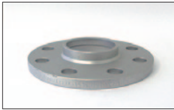
Artikel-Nr./Part-no. 2064640: Radnabenlänge max. 11 mm. Wheel hub length max. 11 mm.
