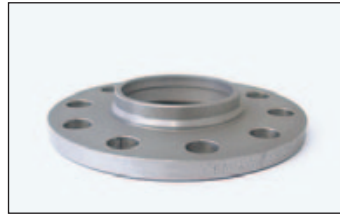
Artikel-Nr./Part-no. 2075725, 2075726: Radnabenlänge max. 12 mm. Wheel hub length max. 12 mm.
