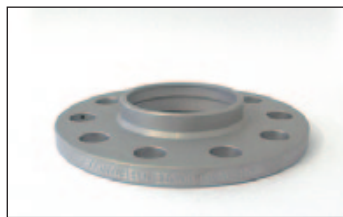
Artikel-Nr./Part-no. 20656710: Radnabenlänge max. 11 mm. Wheel hub length max. 11 mm.
