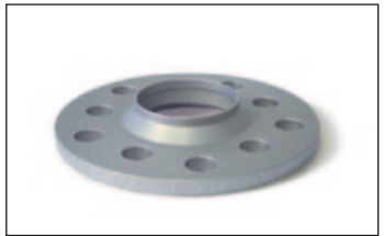
Artikel-Nr./Part-no. 16255570: Radnabellänge max. 13,5 mm. Felgeninnenfase mind. 7x45° Wheel hub length max. 13,5 mm. Inner bavel 7x45°.
