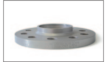
Artikel-Nr./Part-no. 2455668: Radnabenlänge max. 13,5 mm. Felgeninnenfase mind. 4x45° Wheel hub length max. 13,5 mm. Inner bavel 4x45°
