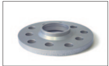
Artikel-Nr./Part-no. 20255570B: Radnabellänge max. 13,5 mm. Felgeninnenfase mind. 5x45° Wheel hub length max. 13,5 mm. Inner bavel 5x45°.
