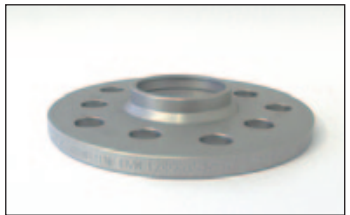
Artikel-Nr./Part-no. 2055571B: Radnabellänge max. 12 mm. Felgeninnenfase mind. 4x45° Wheel hub length max. 12 mm. Inner bavel 4x45°.
