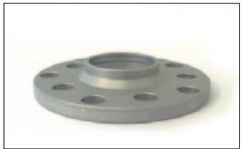
Artikel-Nr./Part-no. 202555712B: Radnabellänge max. 14 mm. Felgeninnenfase mind. 5x45° Wheel hub length max. 14 mm. Inner bavel 5x45°.
